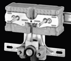
37 578 001 Uniset – pro závěsný bidet • 5 076 Kč nosné úchyty pro bidet, výškově nastavitelné přípojky pro armatury a odpad, odhlučňný EPS-modul pro obezdění
