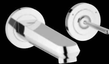
19 968 000 umyvadlová nástěnná, chrom • 7 018 Kč vyložení 170 mm, rozteč 110 mm
