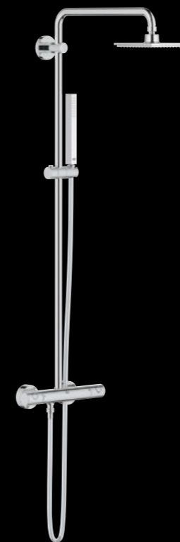
27 932 000 Euphoria Cube • 17 110 Kč set obsahuje: nástěnný termostat s přepínačem, ruční sprchu (27 699 000), hlavovou sprchu (27 705 000), sprchovou hadici 1 750 mm (28 388 000), horizontální otočné sprchové rameno 450 mm, s otočným kloubem, otočný úhel ±25°
