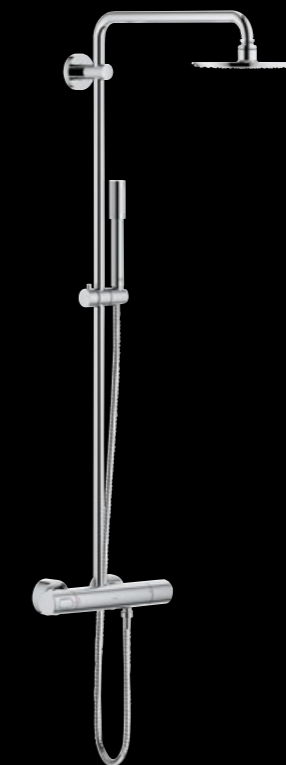
27 032 001 Rainshower • 27 028 Kč set obsahuje: nástěnný termostat s přepínačem, ruční sprchu (27 034 000), hlavovou sprchu 210 mm (28 368 000), kovovou sprchovou hadici 1 750 mm, horizontální otočné sprchové rameno 450 mm, s otočným kloubem, otočný úhel ±20°
