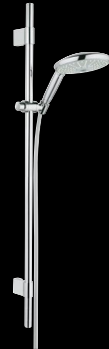
28 770 001 Rainshower • 6 090 Kč ruční sprcha (28 765 000), sprchová tyč 900 mm (28 819 001), hadice 1 750 mm (28 388 000)
